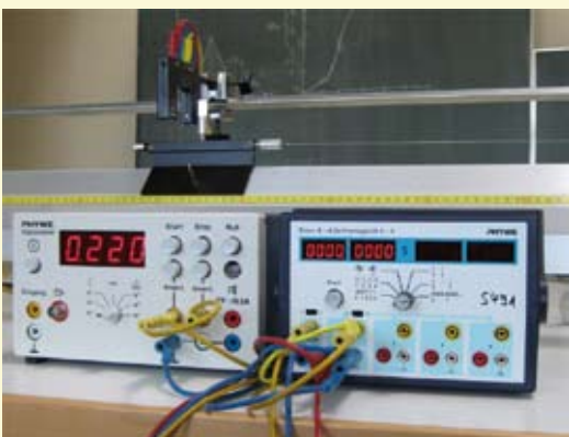
Versuchsaufbau im Physikunterricht
